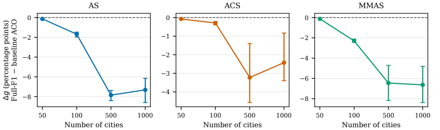
图 3. 主结果: Full-F1 与 baseline ACO 的参考差距之差。误差线为分层 bootstrap 95% 区间。负值支持 Full-F1。图内坐标保留英文。
