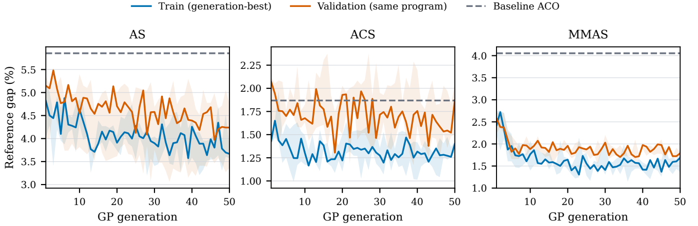
图 4. TSP100 训练与验证曲线。每个运行的训练点是当前代最佳个体在该代新训练批量上的结果。验证点是同一个体在固定 selection 集上的结果。实线为三个独立 GP 运行的中位数。阴影为最小值和最大值。图内坐标保留英文。
